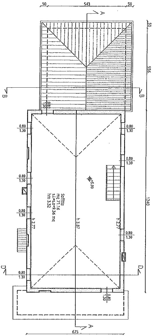
PIANTA PIANO SECONDO
